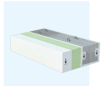
^ Detail skladby nosných a nenosných překladů při tloušťce stěny 500 mm.
